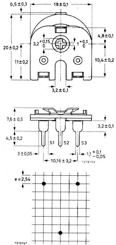
Fig.5 Potentiometer 2322 411 033..
