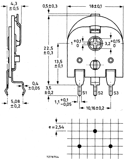
Fig.4 Potentiometer 2322 411 073..
