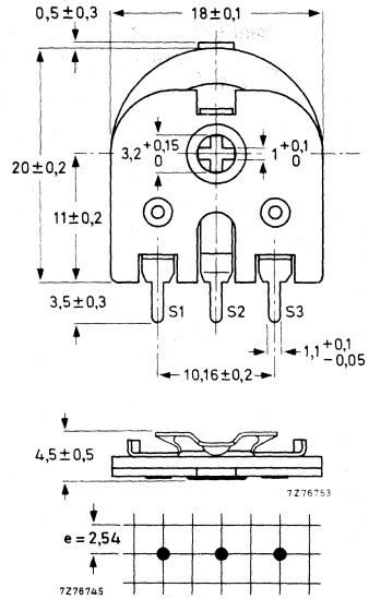
Fig.2 Potentiometer 2322 411 022..
