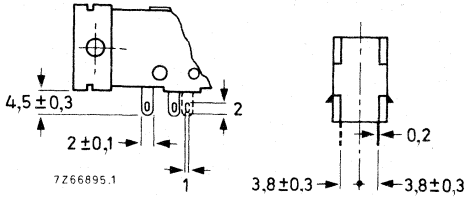
Fig. 3 Solder tags.
