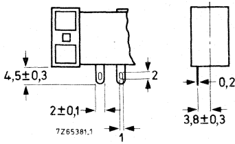
Fig. 3 Solder tags.
