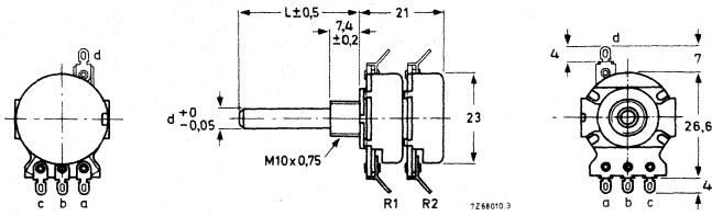
Fig. 2 Tandem potentiometer.
